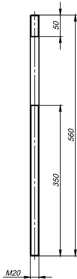
Поз.4 (Шпилька)
